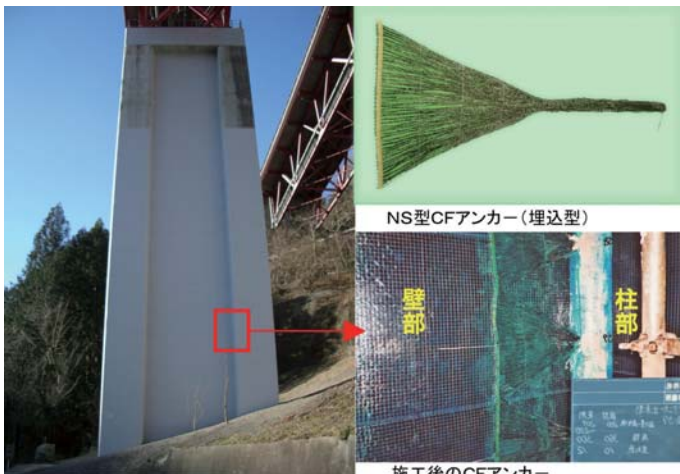
写真2. 土木構造物への適用事例 (中央自動車道・底沢大橋)
